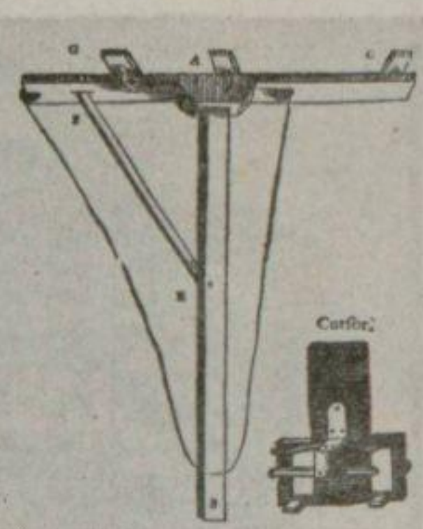
★ Zo moet de sextant er uitzien, die omstreeks 1600 ergens in Friesland is verdwenen.
